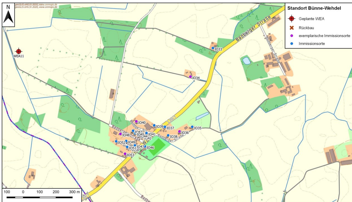
Abbildung 7: Lage der betrachteten Immissionsorte, Detailansicht IO 33-IO 53
