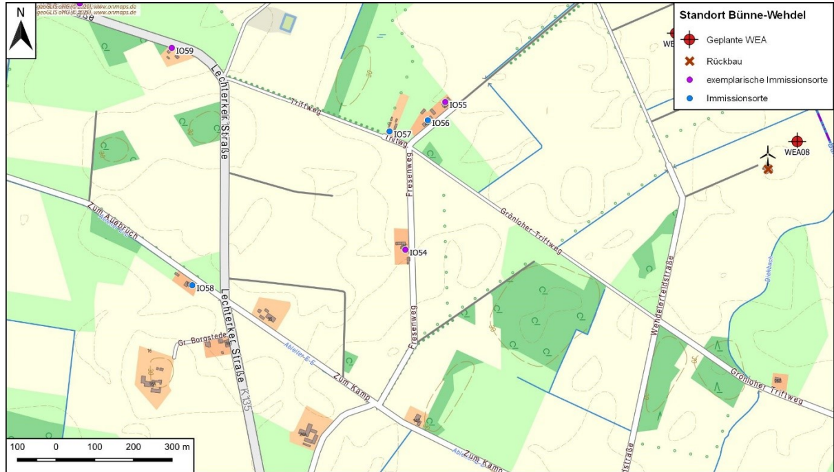
Abbildung 8: Lage der betrachteten Immissionsorte, Detailansicht IO 54-IO 59
