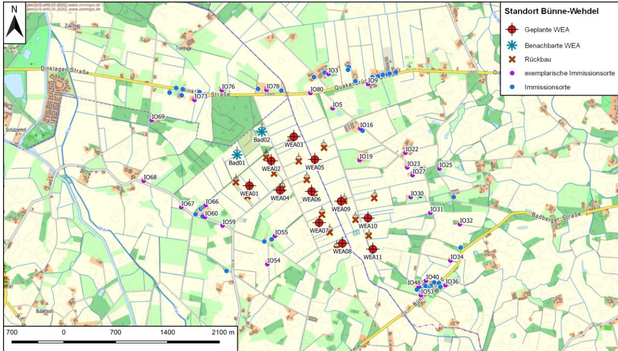
Abbildung 4: Lage der betrachteten Immissionsorte und der WEA am Standort Bünne-Wehdel
