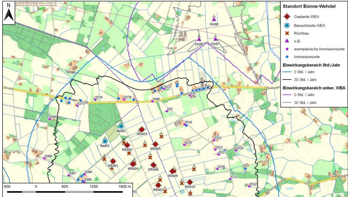
Abbildung A.7: Einwirkungsbereiche der unberücksichtigten WEA und der geplanten WEA
