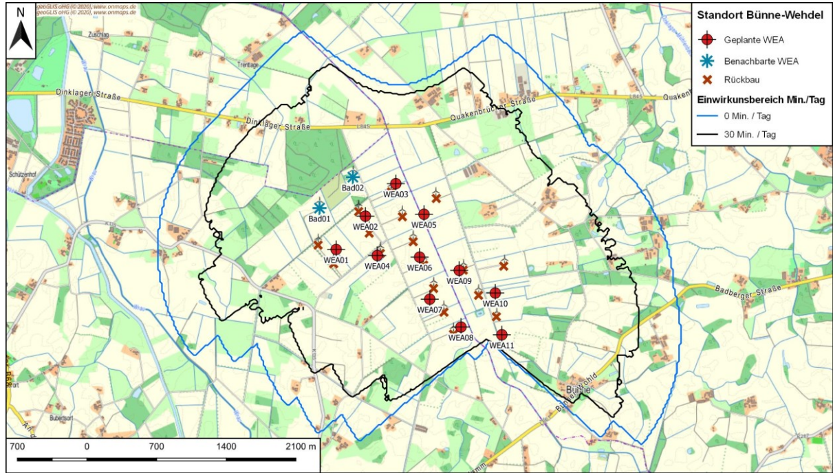
Abbildung 3: Einwirkungsbereich Schattenwurf, Kriterium Minuten pro Tag
