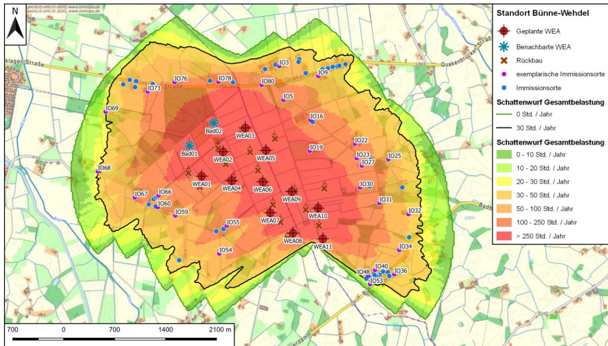
Abbildung 11: Schattenwurf Gesamtbelastung, Kriterium 30 Stunden pro Jahr
