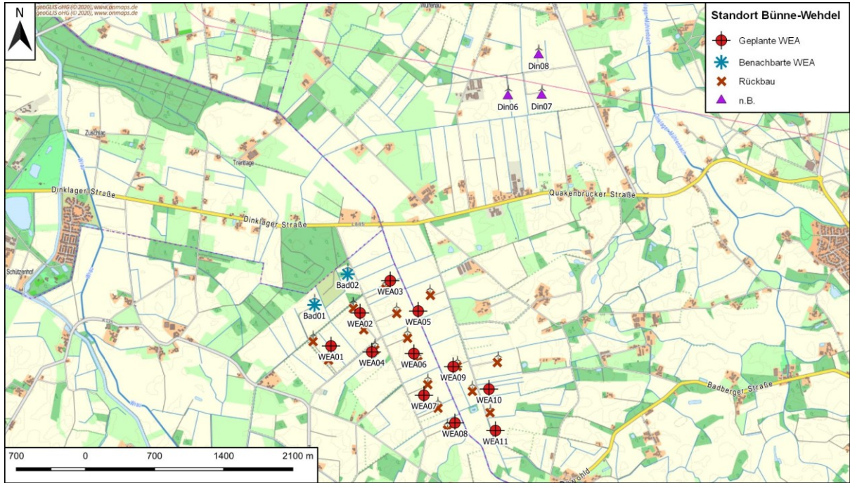
Abbildung 1: Lage der neu geplanten WEA und der benachbart bestehenden WEA am Standort Bünne-Wehdel
