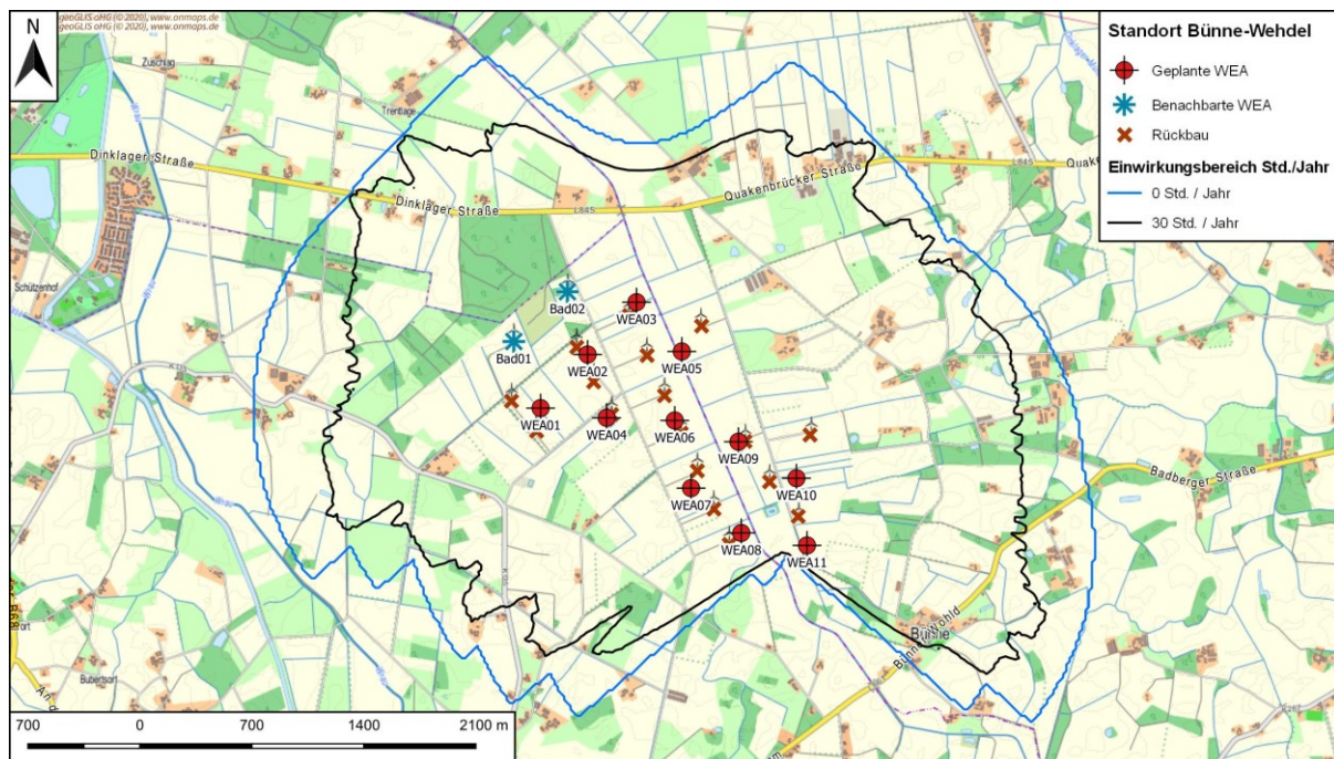
Abbildung 2: Einwirkungsbereich Schattenwurf, Kriterium Stunden pro Jahr
